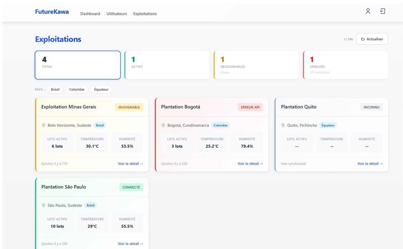
Figure 3 — Liste des exploitations avec filtres de statut et de pays
